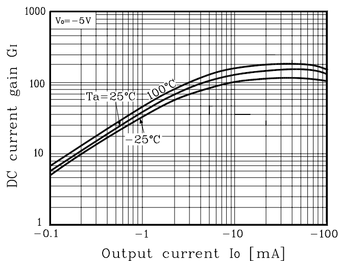
Fig. 4 G_I - I_O
